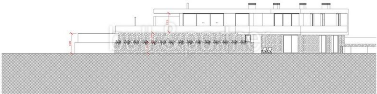
2 Alzado Sur A3-5 | 1:150
