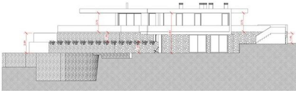
1 Alzado Este A3-4 1:150
